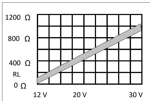
Diagramm RL als Funktion der Betriebsspannung
