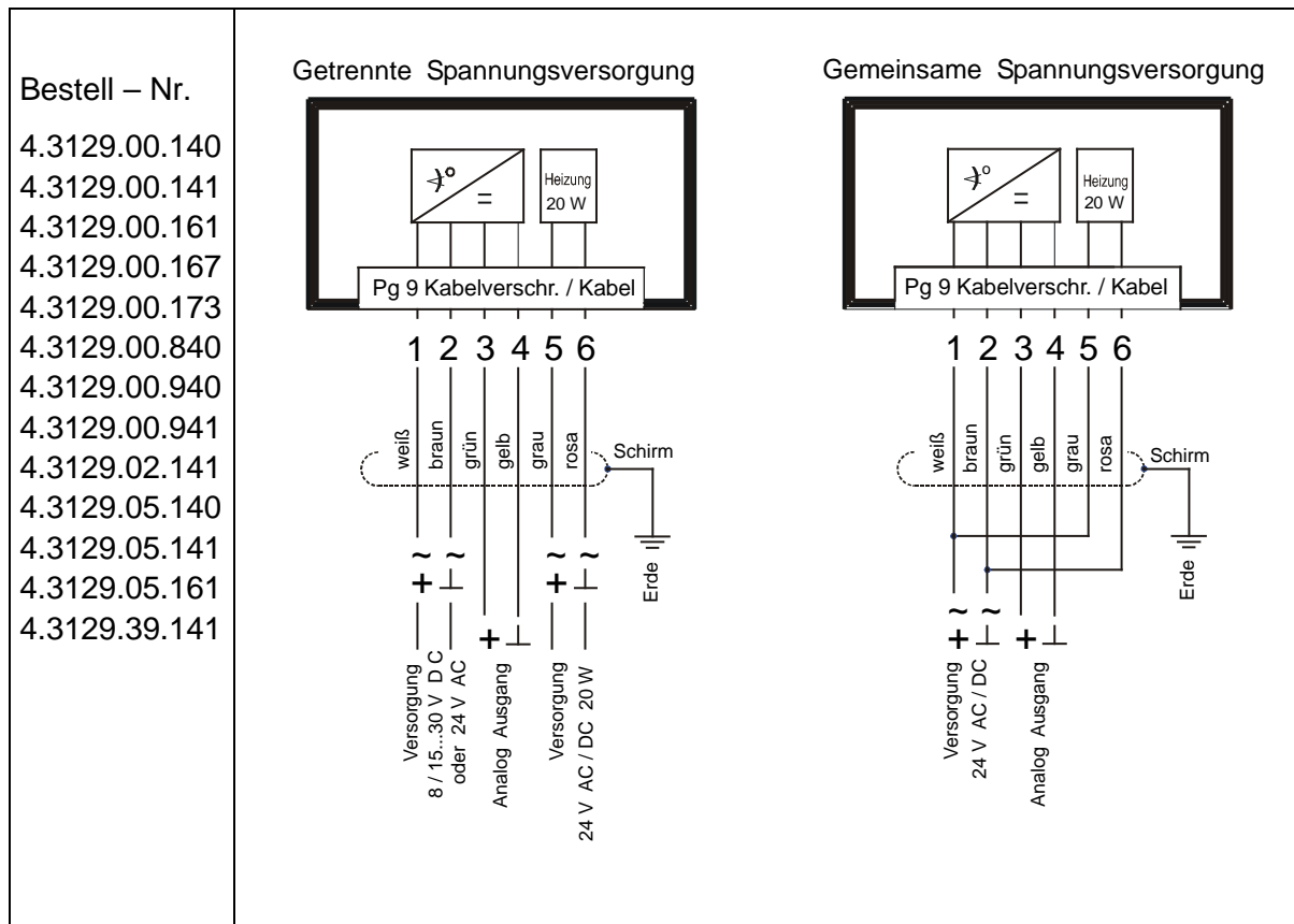
Abbildung 1: Anschlussschaltbild für Ausführungen mit Kabel
