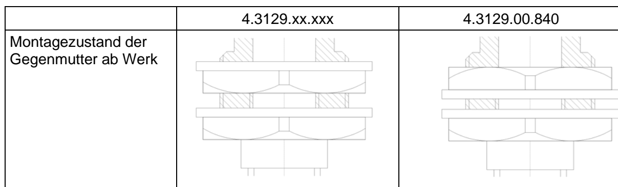
Abbildung 5: Gegenmutter
