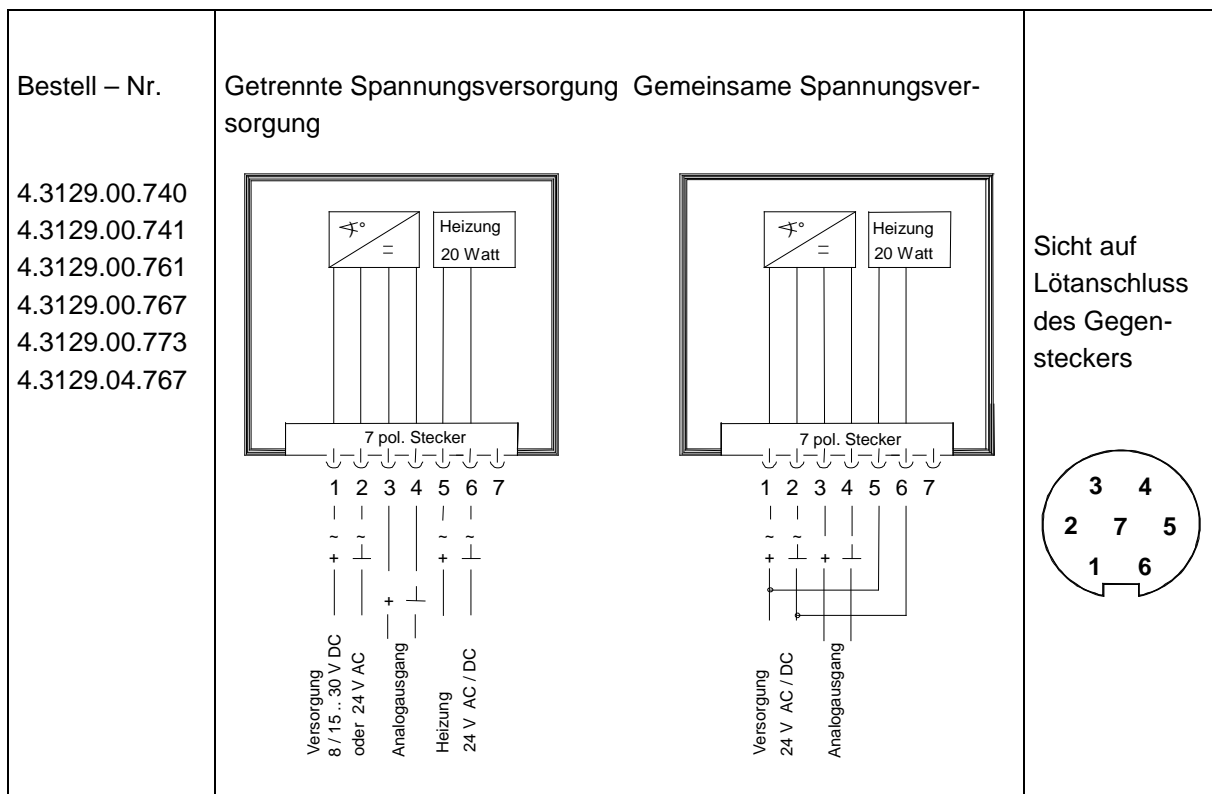
Abbildung 2: Anschlussschaltbild für Ausführung mit Stecker
