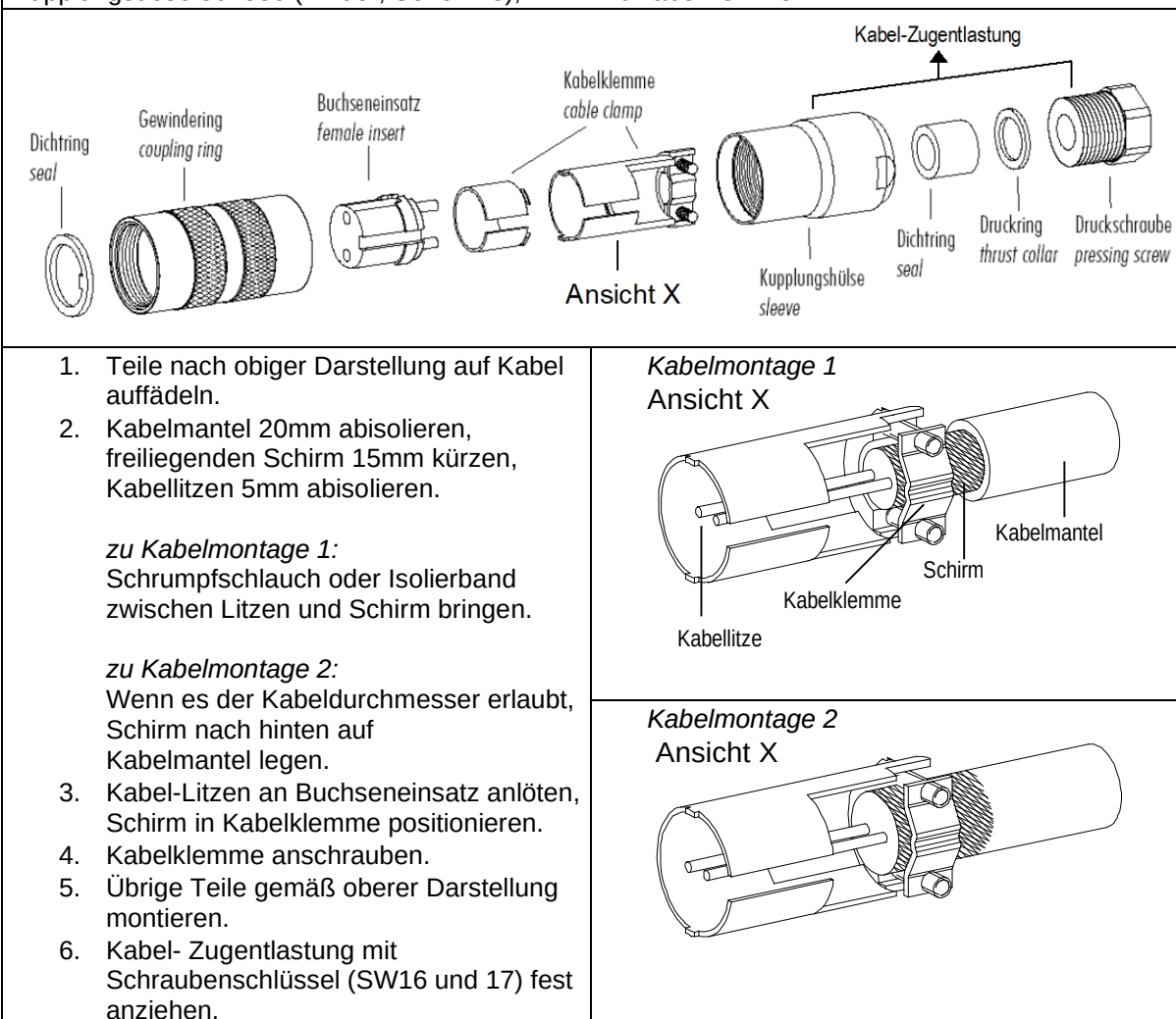
Abbildung 2: Montage Kupplungsdose
